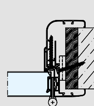
Fissaggio su precassa in legno.
