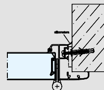
Fissaggio su muro compatto.
