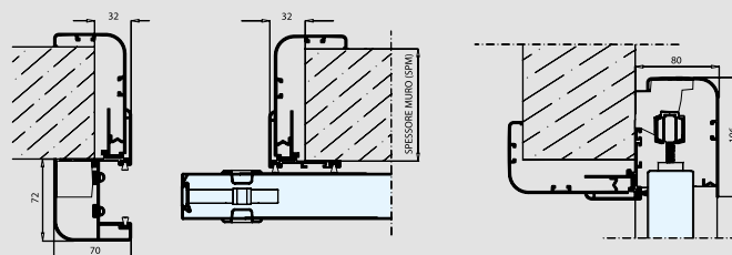
Sezioni apertura scorrevole esterno muro.
