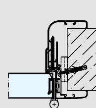
Fissaggio su muro compatto.
