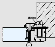
Fissaggio su precassa.
