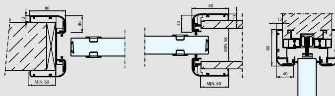
Sezioni apertura scorrevole interno muro.
