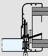
Fissaggio su parete in cartongesso.
